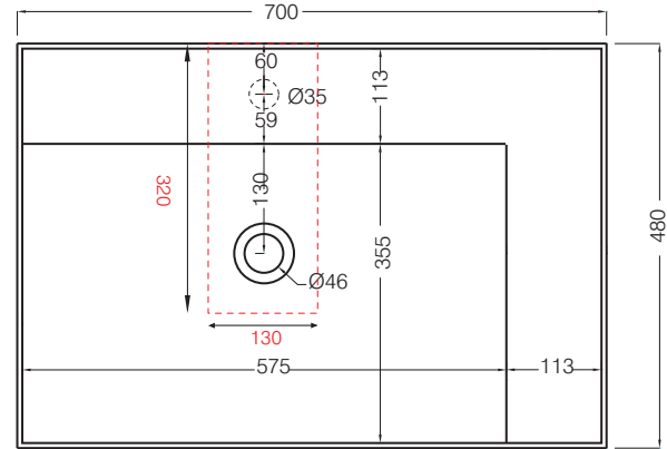
カウンター開口寸法：130×320
