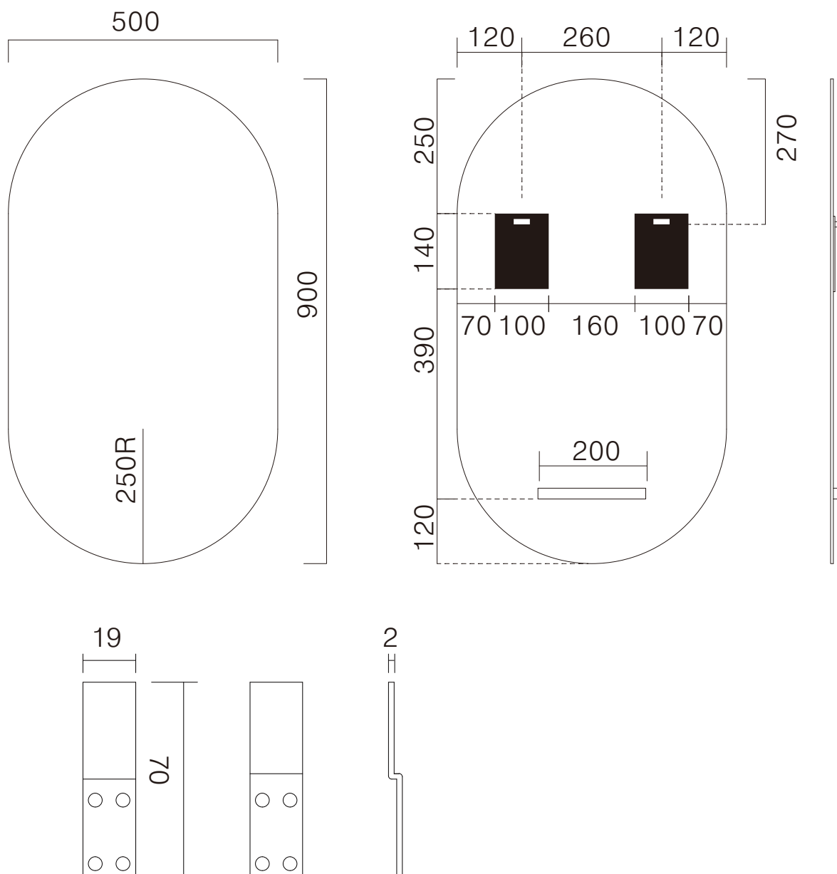
取り付け金具形状
