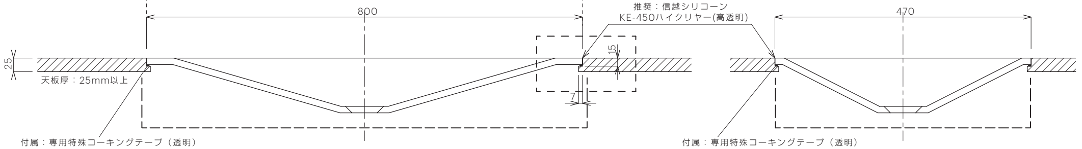
A~A'断面図
